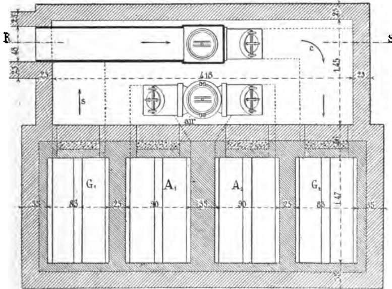
Fig. 143 et 144. — Valve de renversement de fours Siemens.
